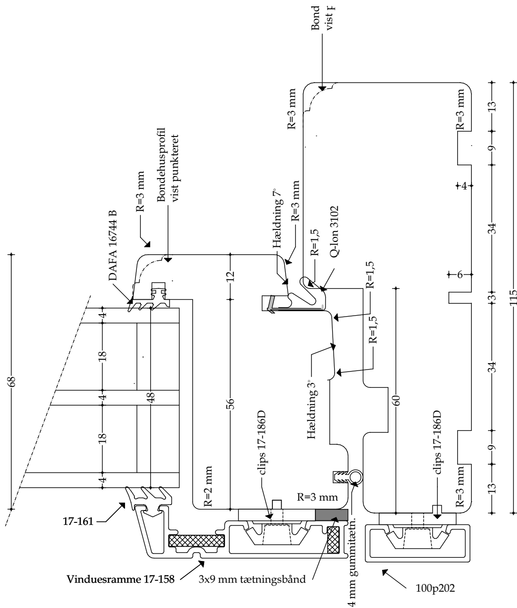
Træ-/alu sidekarm - mål 1:1
