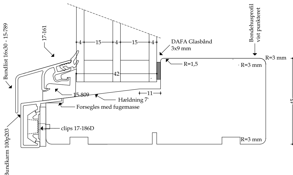
Træ-/alu bundkarm (fastkarm) - mål 1:1
