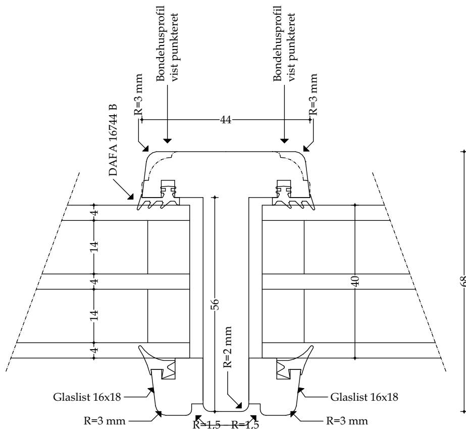
Træ lodret sprosse (lille) - mål 1:1
