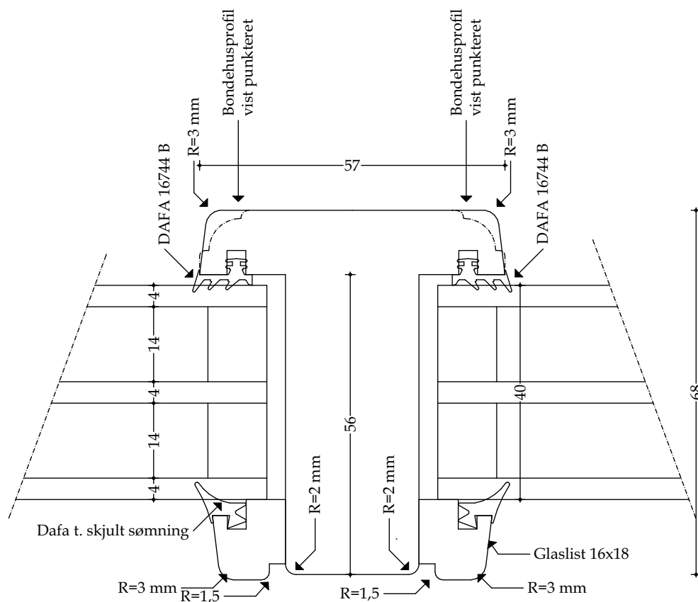
Træ lodret sprosse (stor) - mål 1:1
