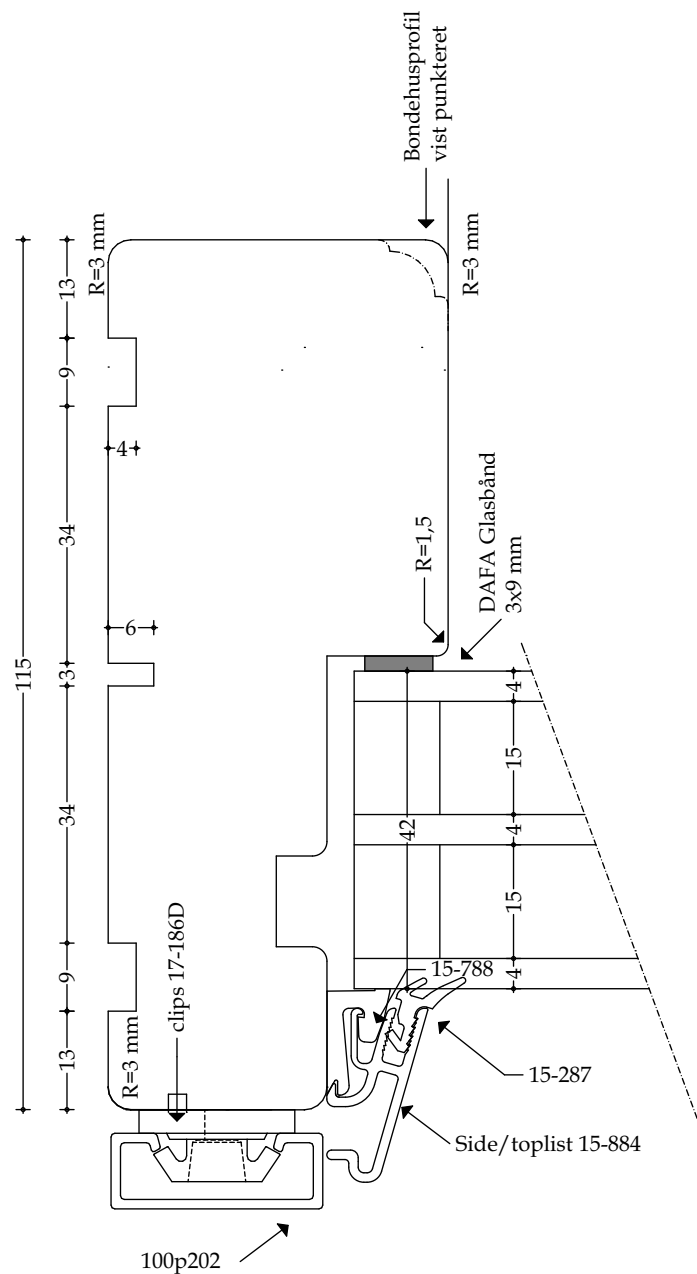
Træ-/alu sidekarm (fast) - mål 1:1
