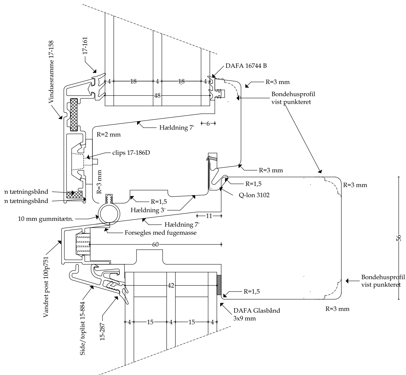
Træ-/alu vandret post med oplukkelig ramme og fastkarm - mål 1:1
