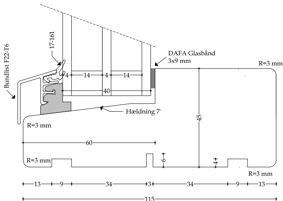
Træ bundkarm (fastkarm) - mål 1:1
