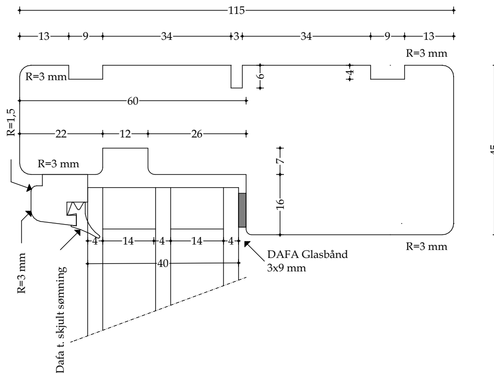
Træ topkarm (fastkarm) - mål 1:1
