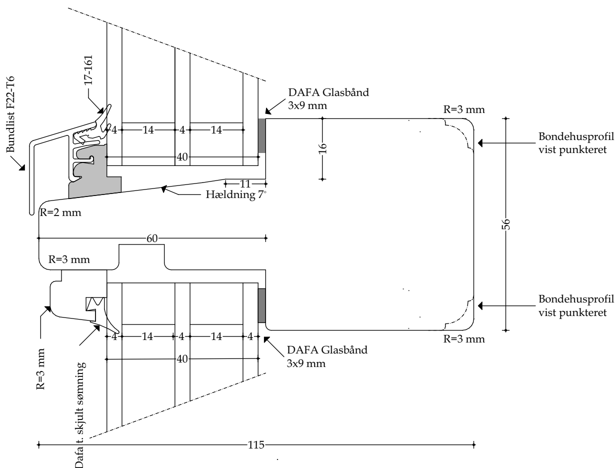
Træ vandret post ved fastkarm - mål 1:1
