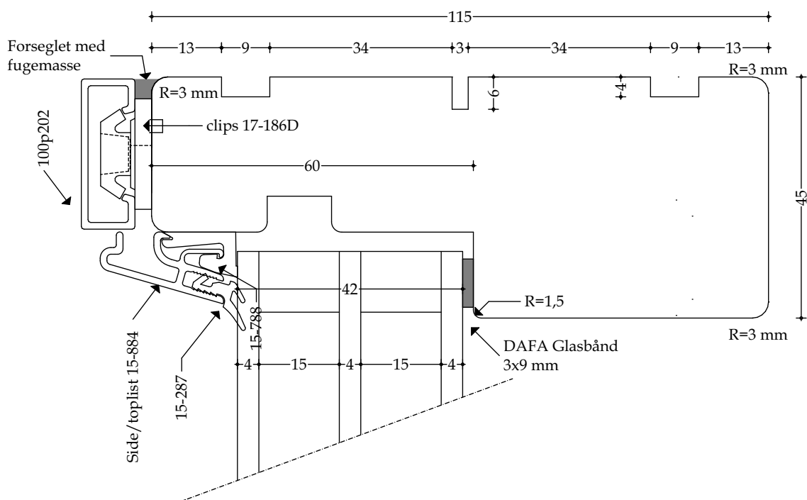
Træ-/alu topkarm (fastkarm) - mål 1:1
