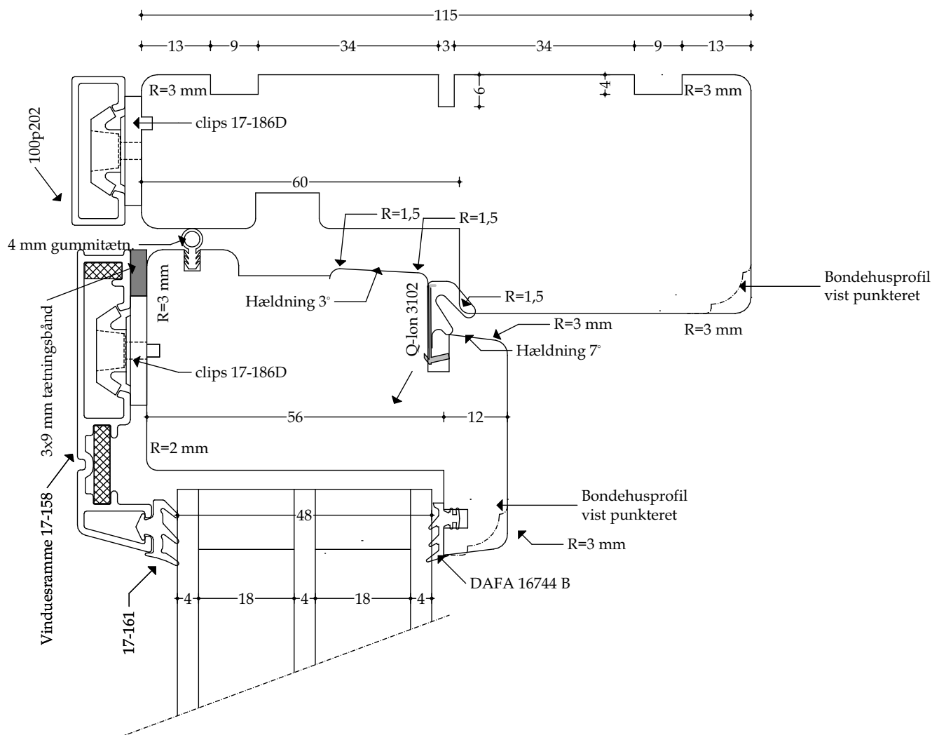
Træ-/alu topkarm - mål 1:1
