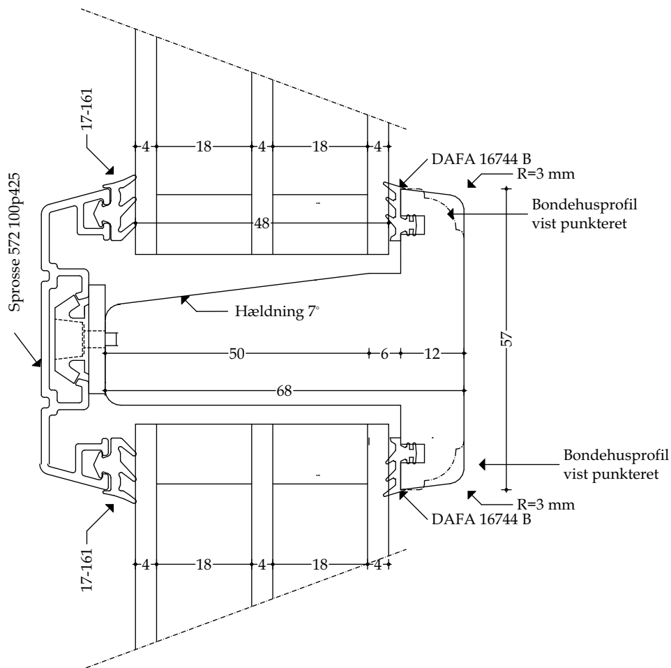
Træ-/alu vandret sprosse (stor) - mål 1:1
