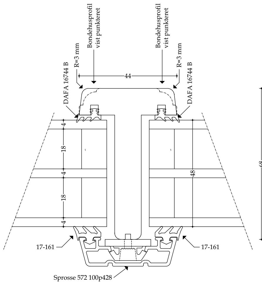
Træ-/alu lodret sprosse (lille) - mål 1:1
