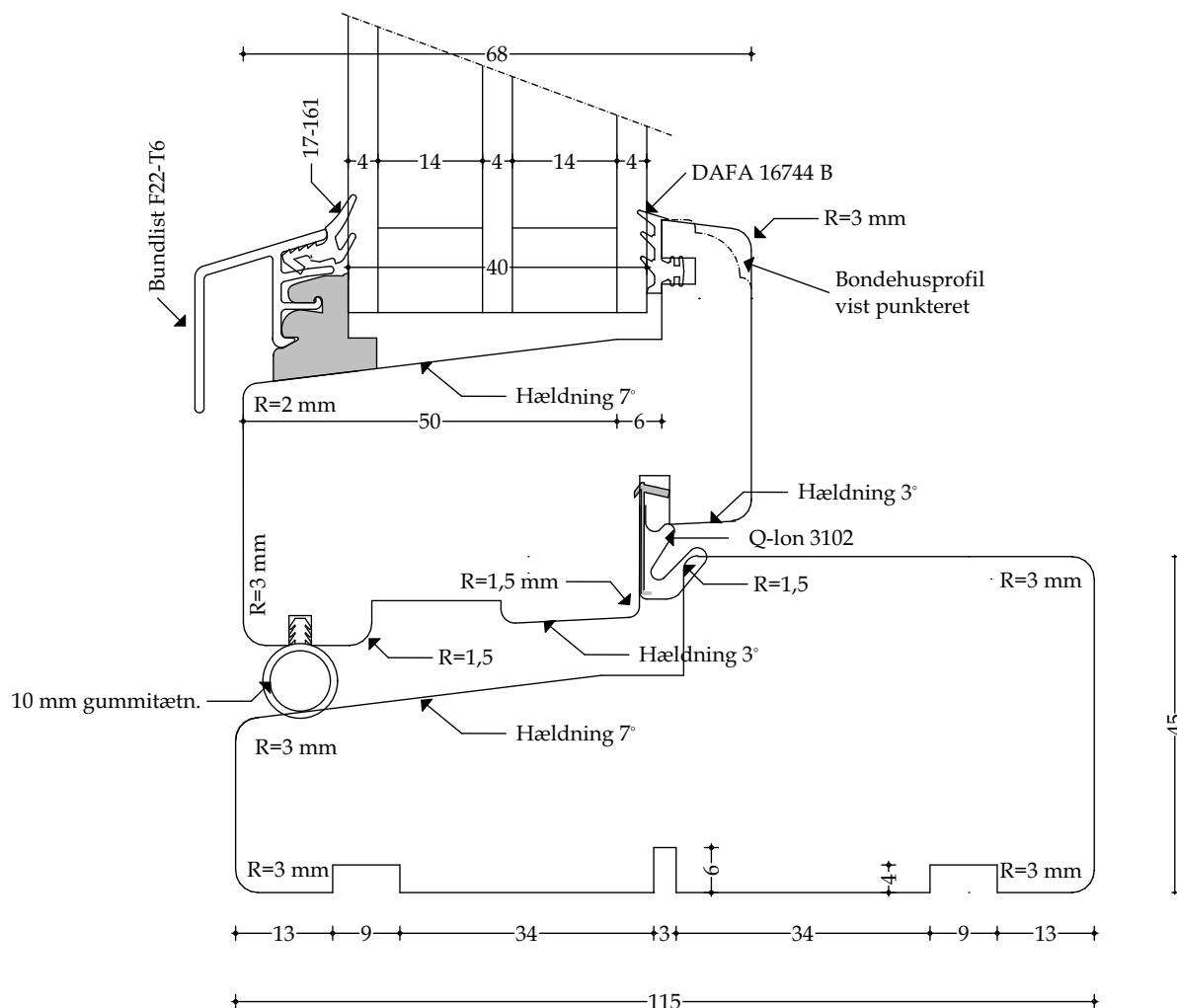
Træ bundkarm ved oplukkelig ramme - mål 1:1
