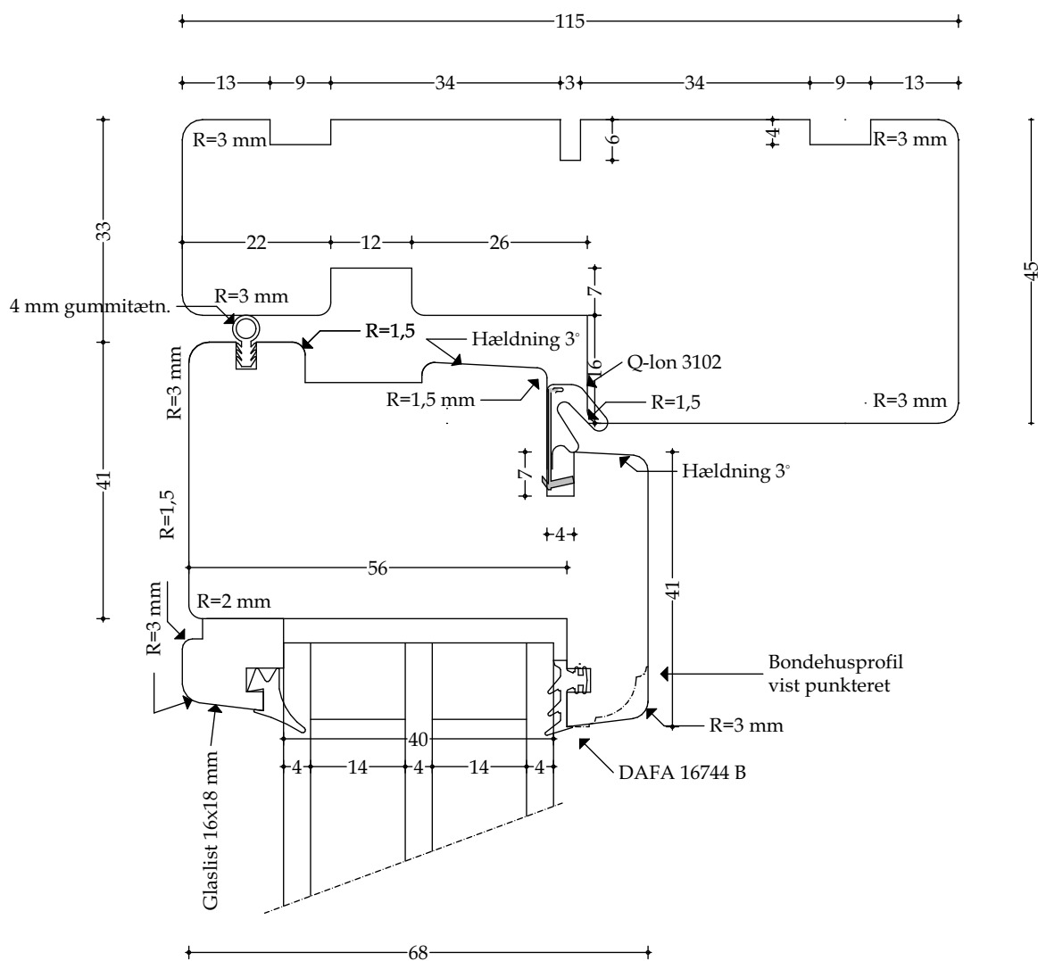
Træ topkarm - mål 1:1
