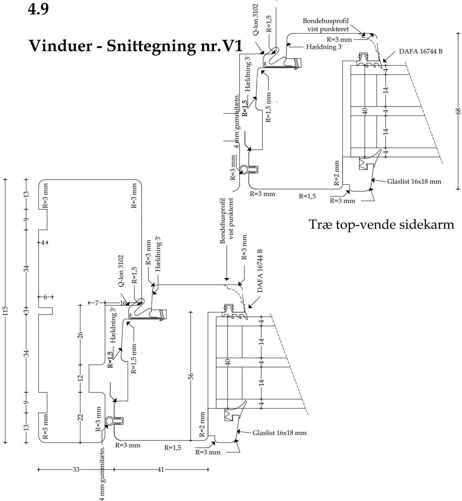
Træ sidekarm - mål 1:1
