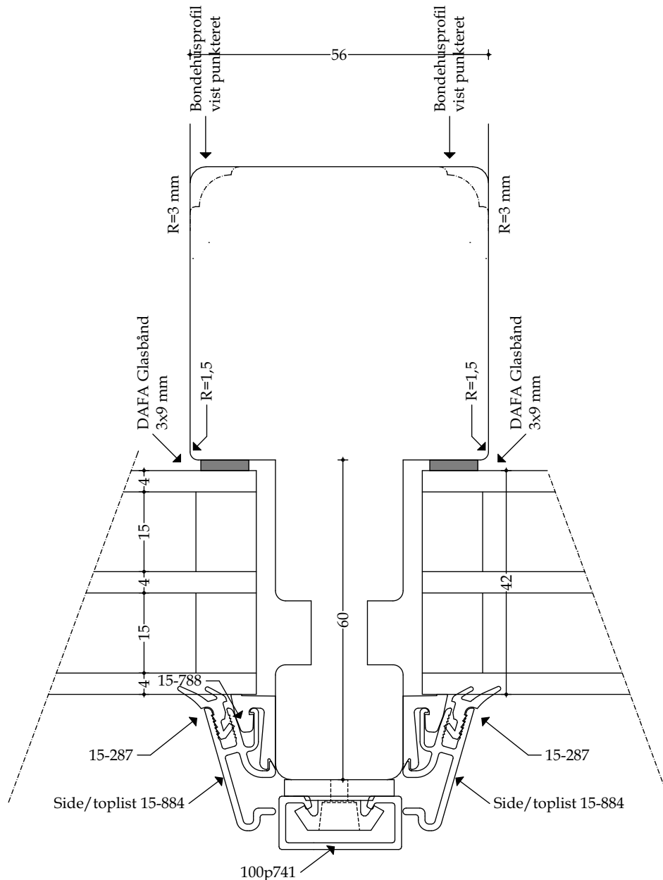
Træ-/alu lodret post i fastkarm - mål 1:1
