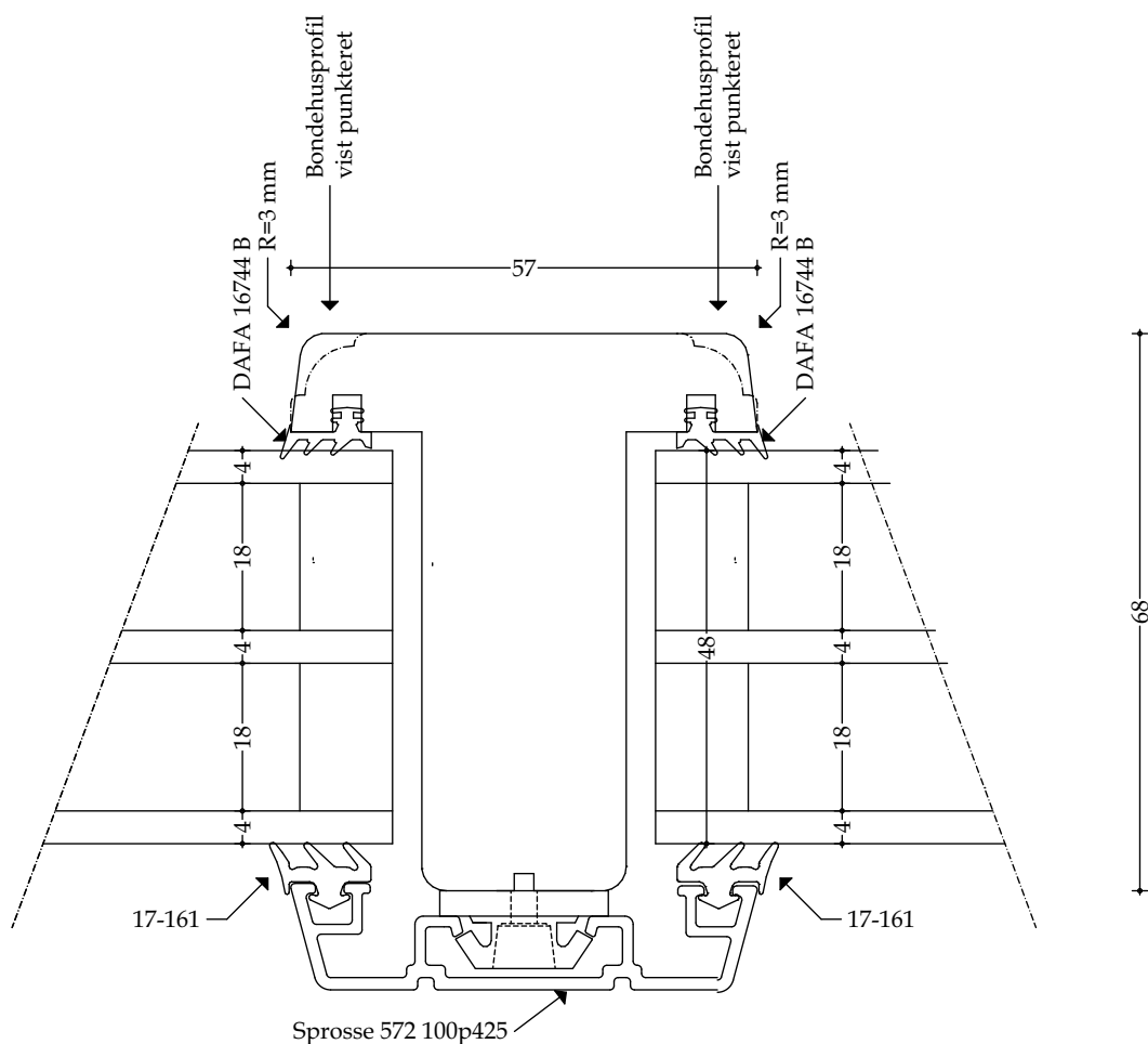
Træ-/alu lodret sprosse (stor) - mål 1:1
