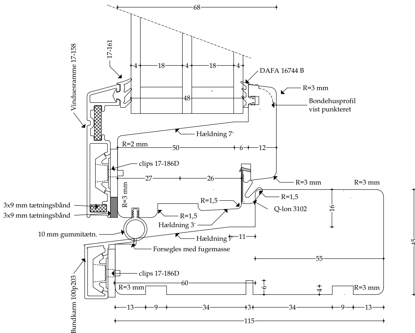
Træ-/alu bundkarm - mål 1:1
